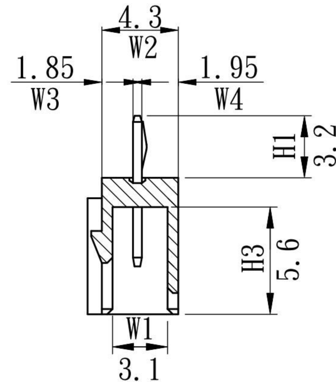
A-A Section
