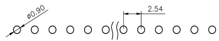
P.C.B LAYOUT
