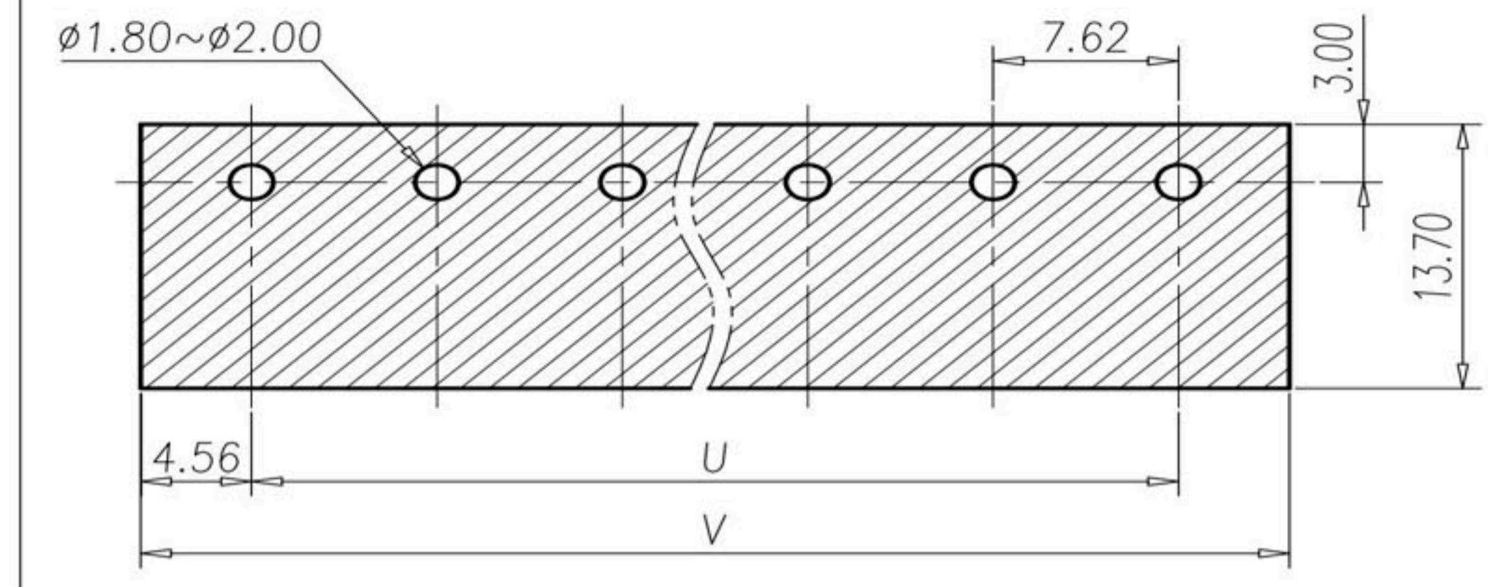
P.C.B. LAYOUT(REF)
