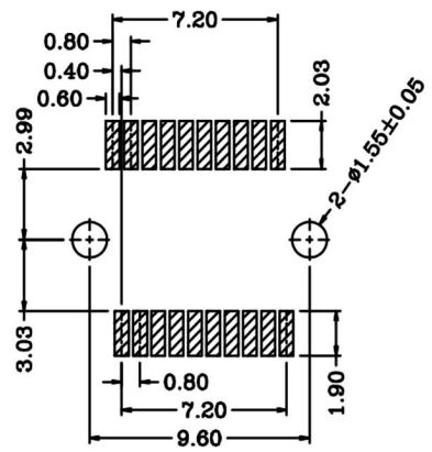
P.C.Board Layout
