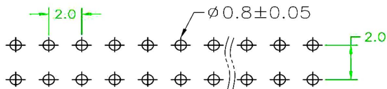
P.C.B LAYOUT
