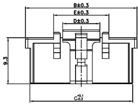
6X2~20X2 PIN
