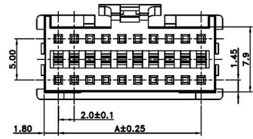
6X2~20X2 PIN
