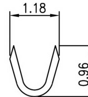
A-A SECTION
